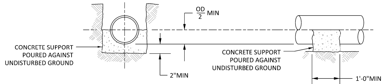
SECTION A-A
